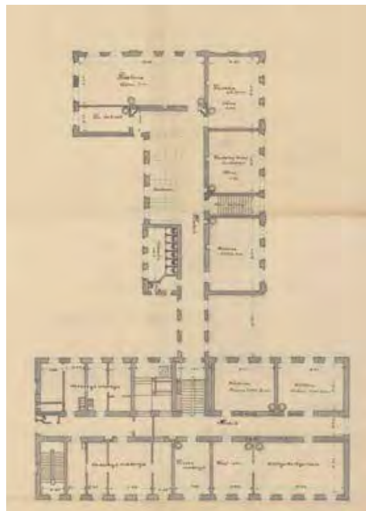
Floris I. nadstropja kočevske gimnazije, 1929 Slovenski šolski muzej
